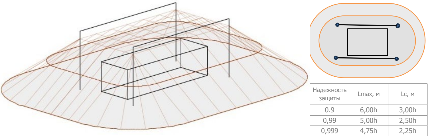
Расчет зоны молниезащиты двойного тросового молниеприемника
