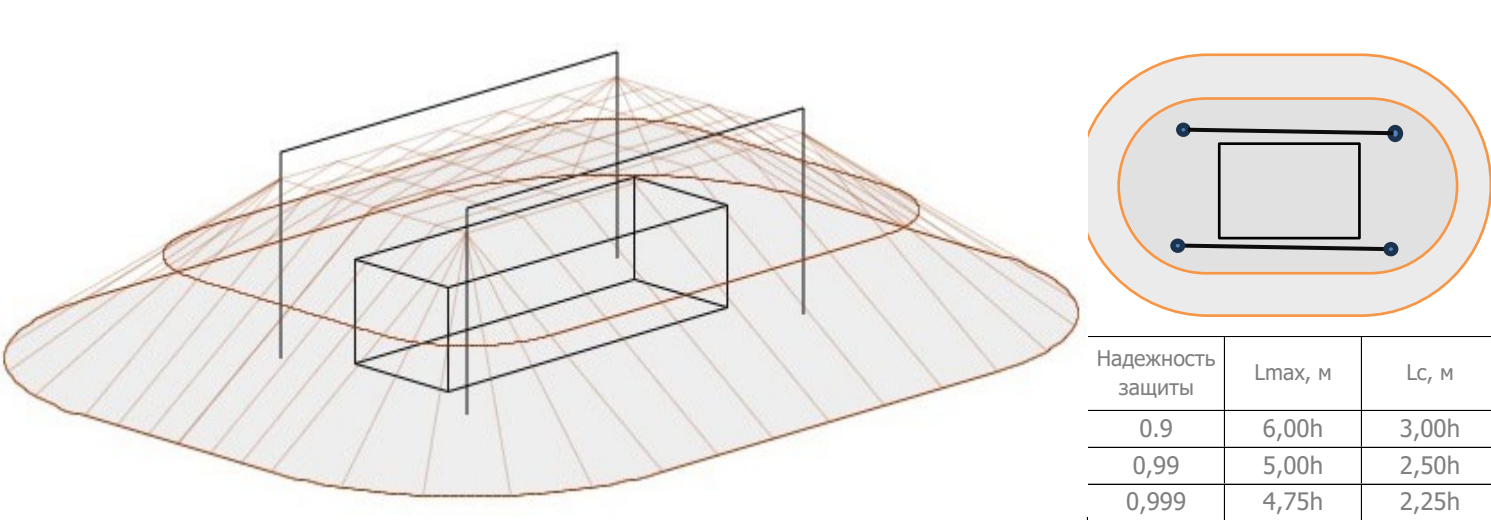
Расчет зоны молниезащиты двойного тросового молниеприемника
